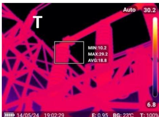
Gambar 5 Hasil Thermovisi Phasa T
